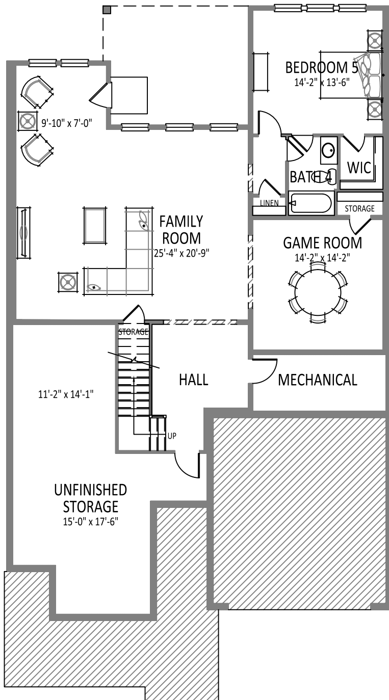
OPTIONAL BASEMENT PLAN
