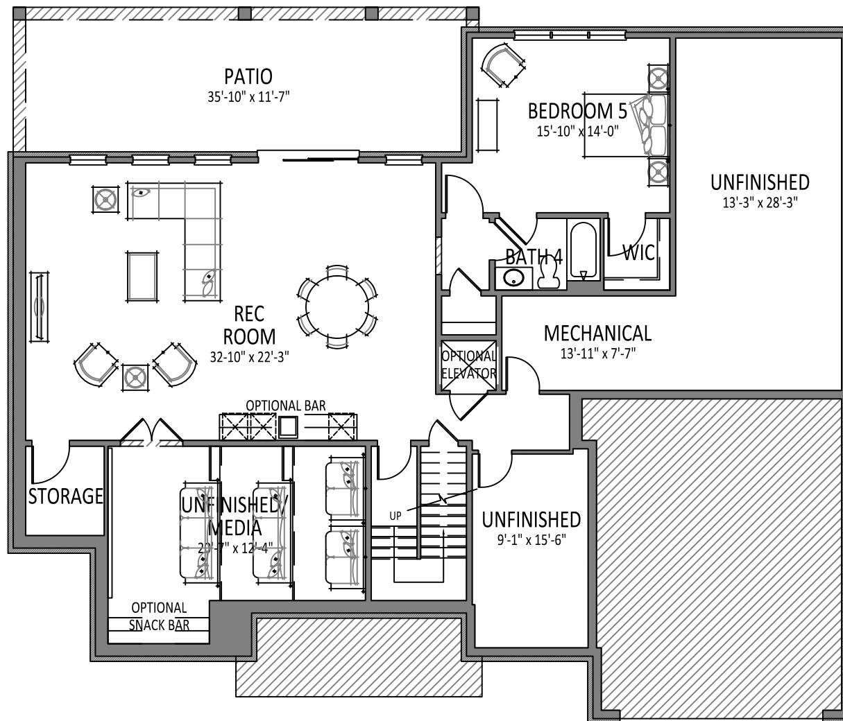
OPTIONAL BASEMENT PLAN
