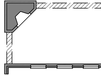
OPTIONAL EXTERIOR FIREPLACE
