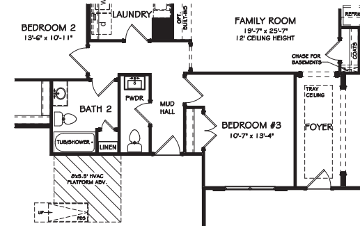
Optional 3rd Bedroom in lieu of Study
