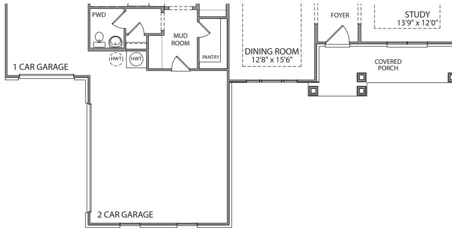
ELEVATION B
